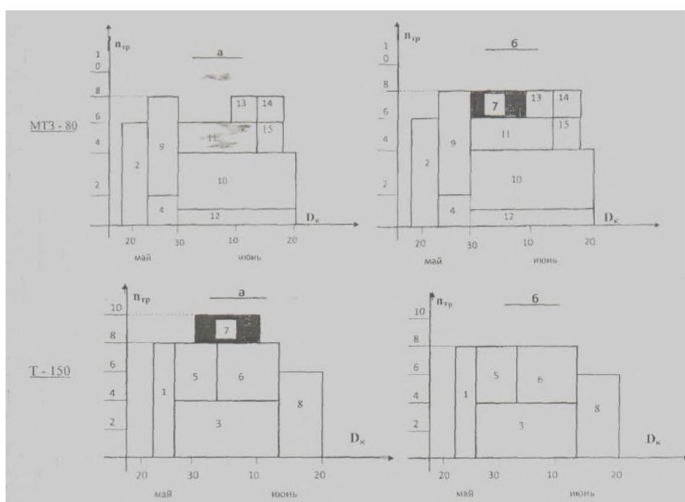
Рис.6. II способ, МТЗ-80 а) до корректировки б) после корректировки
