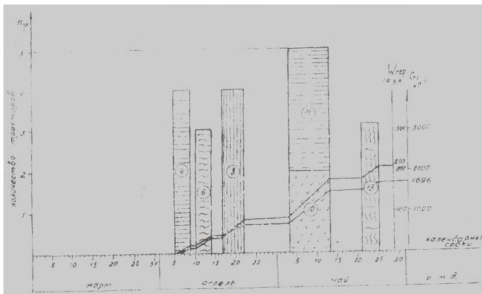
Рис.2. График загрузки тракторов МТЗ 80
