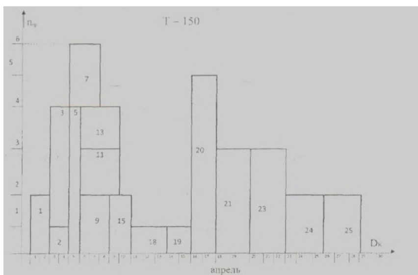
Рис. 3. Графики машиноиспользования (загрузки трактора)
