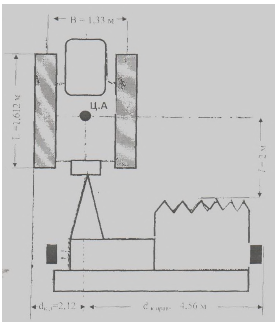
Рис.9. Кинематические параметры силосоуборочного агрегата
