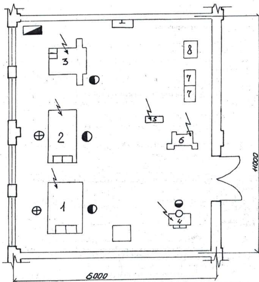
План участка
